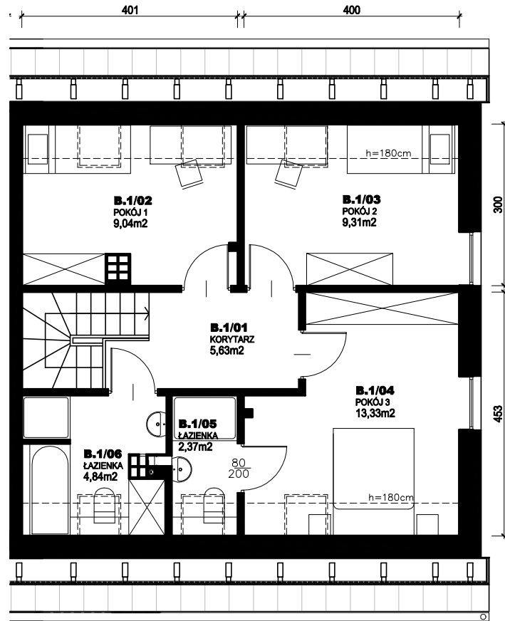
RZUT PODDASZA
